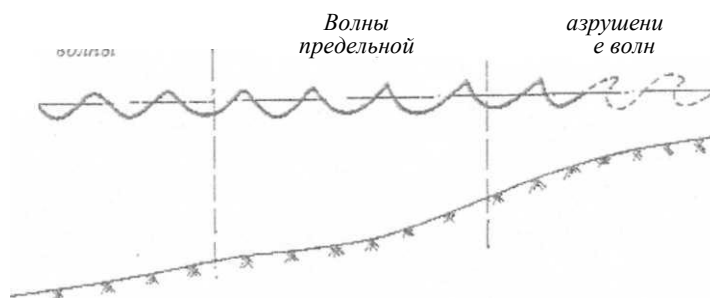
Рис. 6.8. Залежність профіля хвильного рішення рівняння Уизема від глибини [23]
